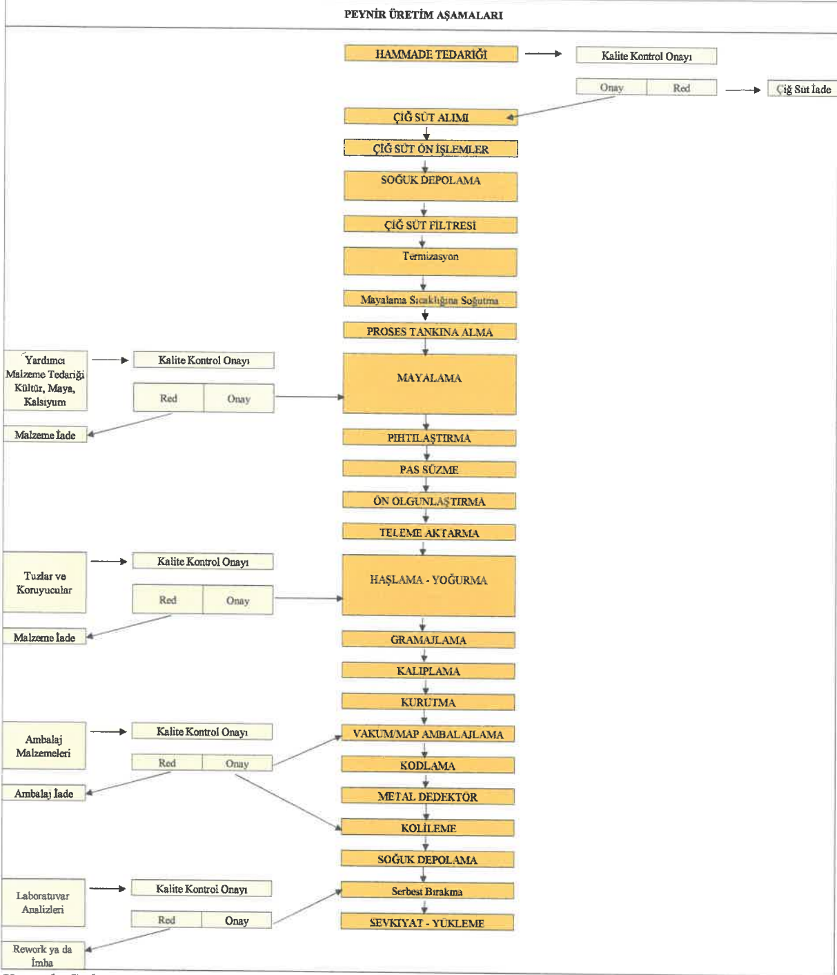
Şekil 1: Üretim Aşamaları Hakkında Akış Şeması
